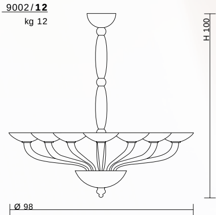
lampadario a 12 luci, twelve light chandelier, Lüster zwölfflammig, lustre à douze lampes
