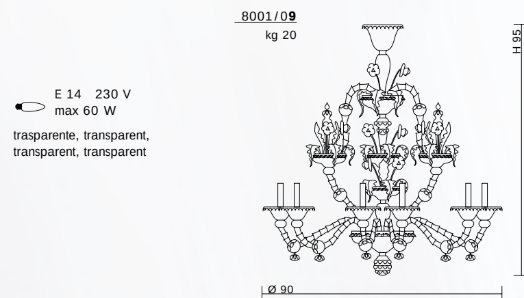
lampadario a 9 luci, nine light chandelier, Lüster neunflammig, lustre à neuf lampes
