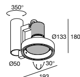
CLUB S H30 A 284 20 1130 A E27Ls / 230-240V / 50-60Hz 1 x QPAR30 75W
