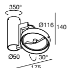
CLUB S 1111 T50 A 284 21 1111 A G53 / 230-240V / 50-60Hz / TE 1 x QR-LP111 35-50W
