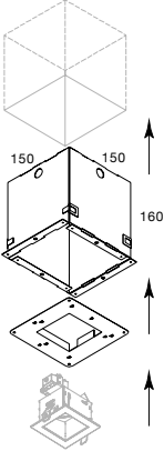
ARTUUR 180 / 180 OK CONCRETE BOX 202 25 18 0,4
