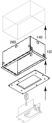
ARTUUR 145 / 235 / 245 CONCRETE BOX 202 25 28 0,4
