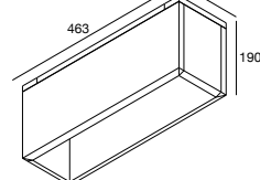
MINIGRID IN ZB 4LINE H20 / RA BOX 202 70 98 14L
